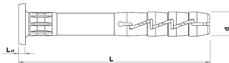
FX-..C.. sleeve
