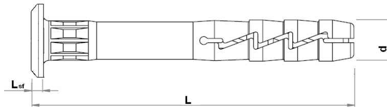
FX-..K.. sleeve
