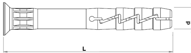
FX-..L.. sleeve
